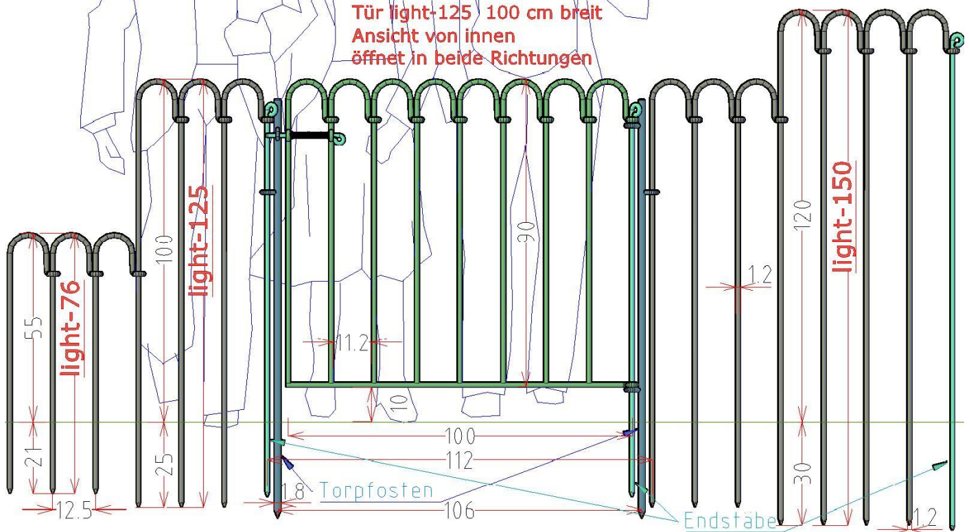
Zeichnung von unseren verschiedenen Steckzäunen Modell light mit Tür light-125-... 100 cm breit.
